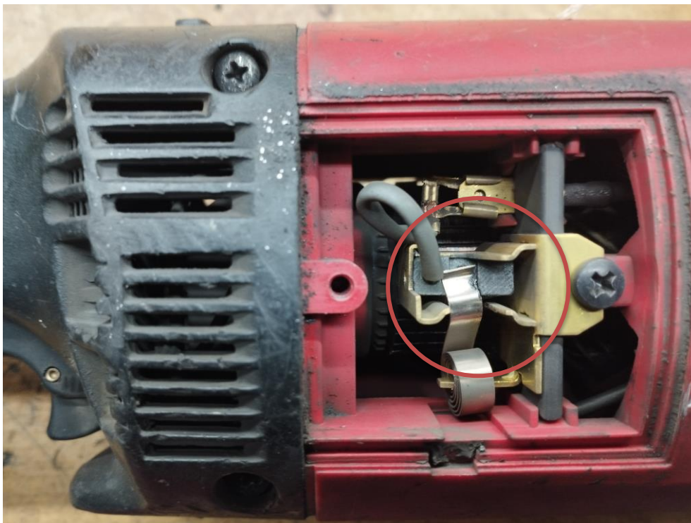
Obr.1 Použitie neoriginálnych kief
