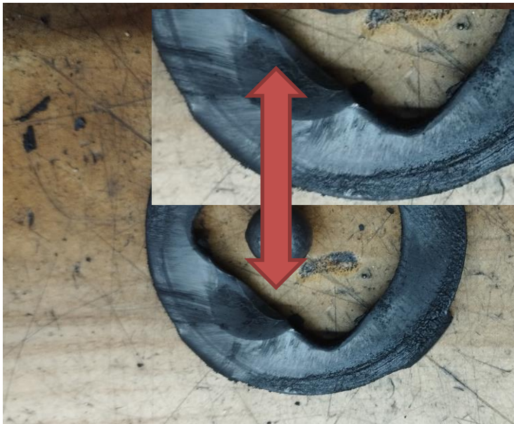
Obr.2 Opatrebenie podložky guličky
